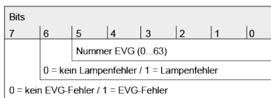
Bild 15: Telegrammaufbau 1-Byte-Fehlerstatus
