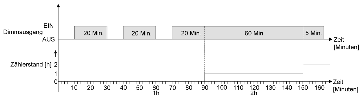
Bild 59: Funktionsweise des Betriebsstundenzählers (am Beispiel gezählter Stunden)
