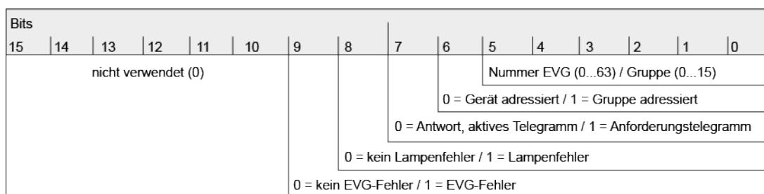
Bild 16: Telegrammaufbau 2-Byte-Fehlerstatus
