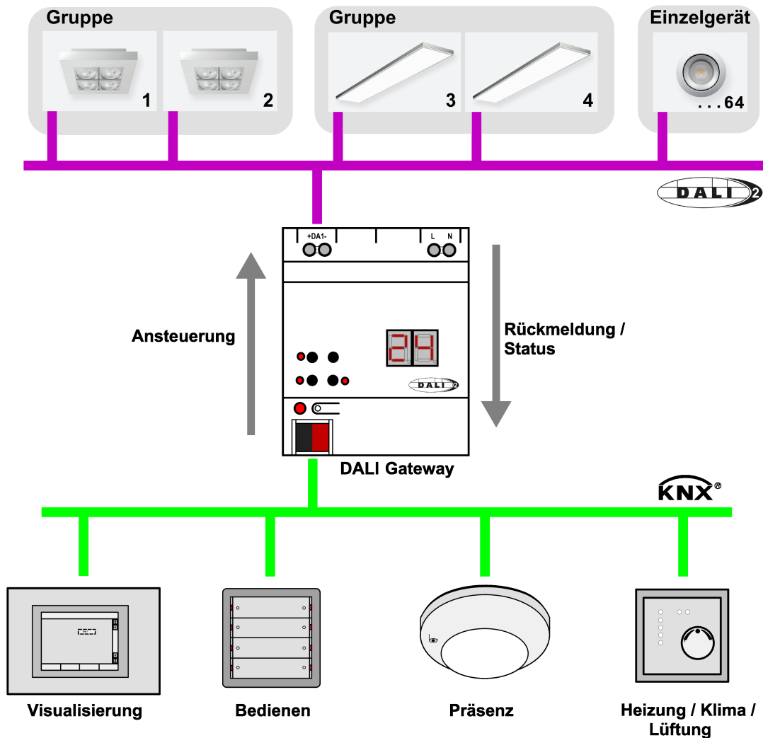
Bild 3: Prinzipübersicht einer KNX DALI Systemanbindung
