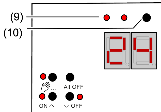
Bild 12: Bedienfeld DALI Gateway 2fach
