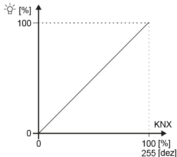
Bild 21: Lineare Dimmkennlinie am Ausgang eines Betriebsgeräts (relativer Lichtstrom [%] abhängig vom 8-Bit-KNX Datenwert [0...255])
